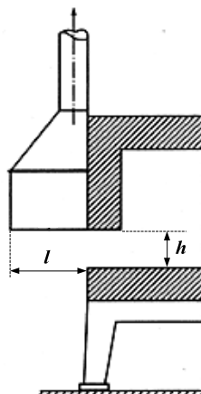
Рис. Вытяжной зонтик-козырек
