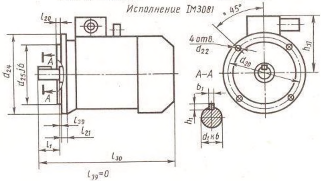
Рис. 1.3 Электродвигатели серии АИР
